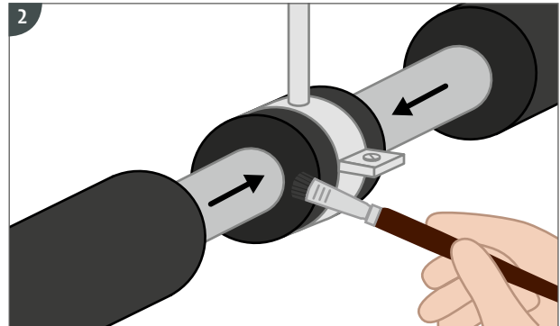
Kälte-Rohrschelle und Rohrdämmung mit Kleber versehen, ablüften lassen und zusammenfügen.
