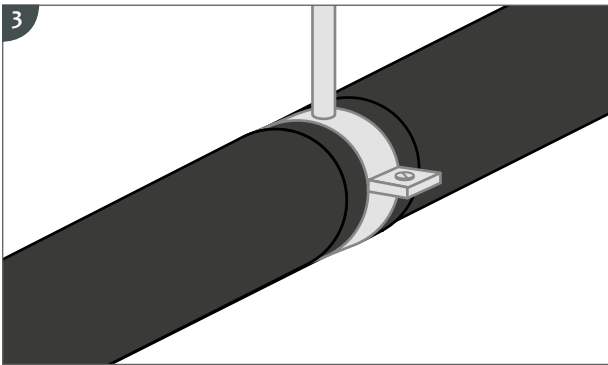
Fertig gedämmte Leitung.
