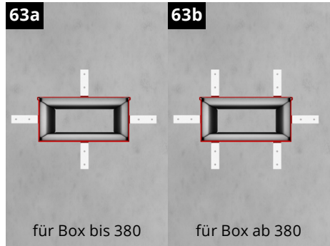
63a für Box bis 380 63b für Box ab 380 Winkel befestigen Winkel am Boxenrand andrücken. (Lieferumfang: 4 bis 6 Winkel je nach Boxengröße)
