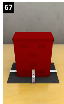
67 FST-Kombibox SB befestigen FST-Kombibox SB auf Schalungsbrett schrauben oder nageln.
