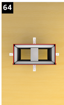
64 Prüfen Mitgelieferten Hartschaumblock mittig anordnen, oben und unten die Schaumplatten. Dadurch kein Verformen der FST-Kombibox beim Vergießen des Ortbetons.
