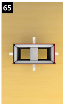
65 Prüfen Mitgelieferten Hartschaumblock mittig anordnen, oben und unten die Schaumplatten. Dadurch kein Verformen der FST-Kombibox beim Vergießen des Ortbetons.
