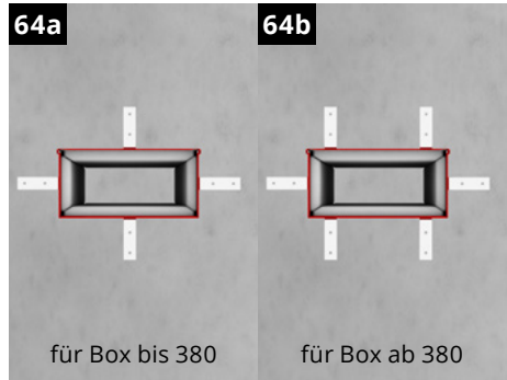
64a 64b für Box bis 380 für Box ab 380 Winkel befestigen Winkel am Boxenrand andrücken. (Lieferumfang: 4 bis 6 Winkel je nach Boxengröße)
